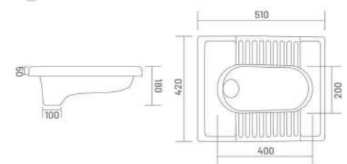
CT PAN - 20" Pan 20" x 17" x 7"
